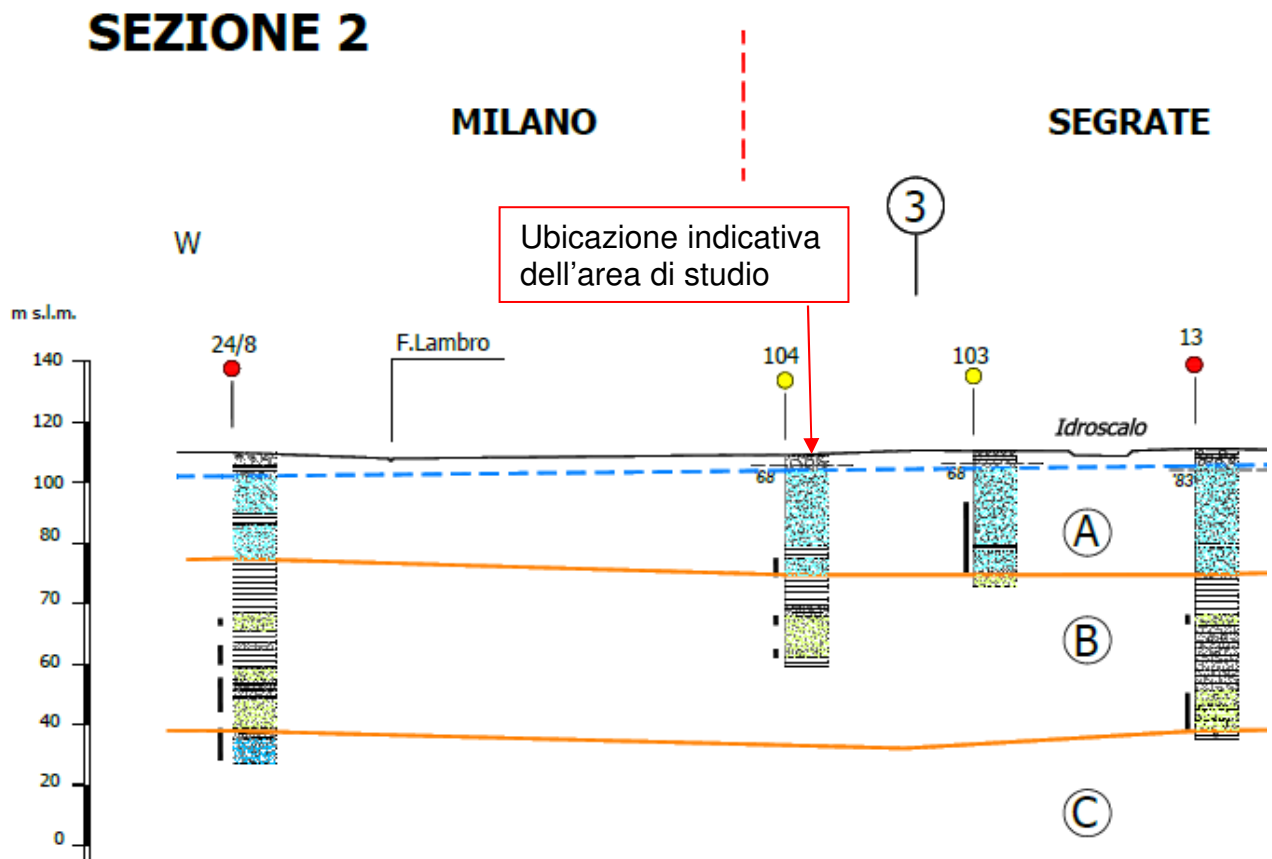
Fig. 7a – Sezione 2 di riferimento
