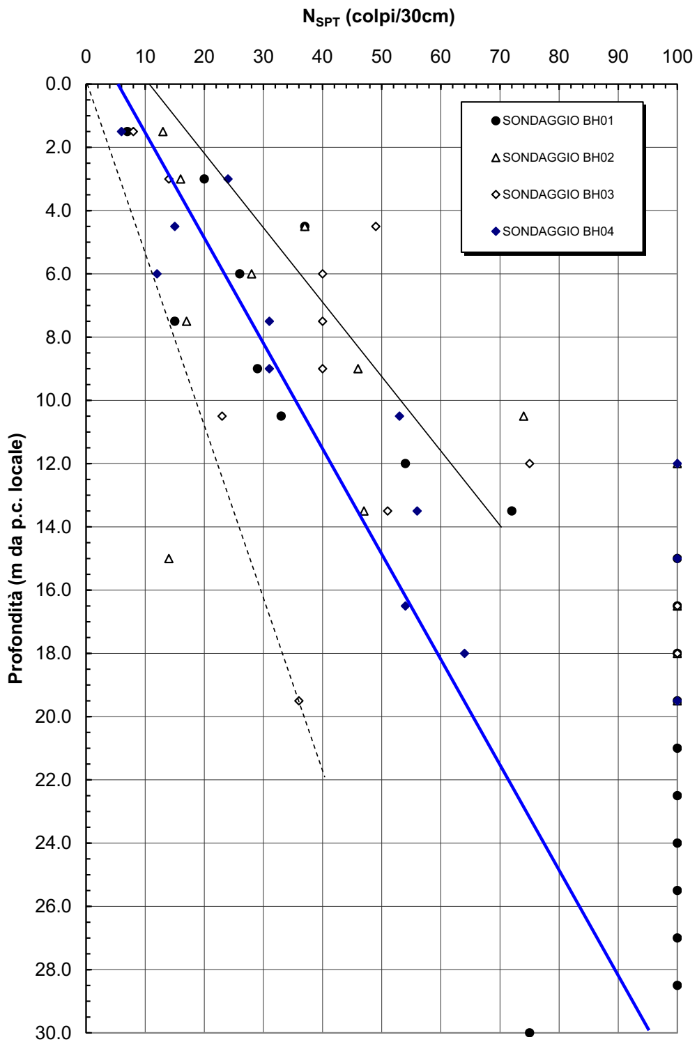
Figura n. 4.2 | Prove SPT - Campagna di indagine 2011
