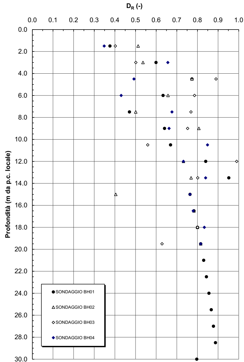
Figura n. 4.4 | Densità relativa da SPT - Campagna di indagine 2011
