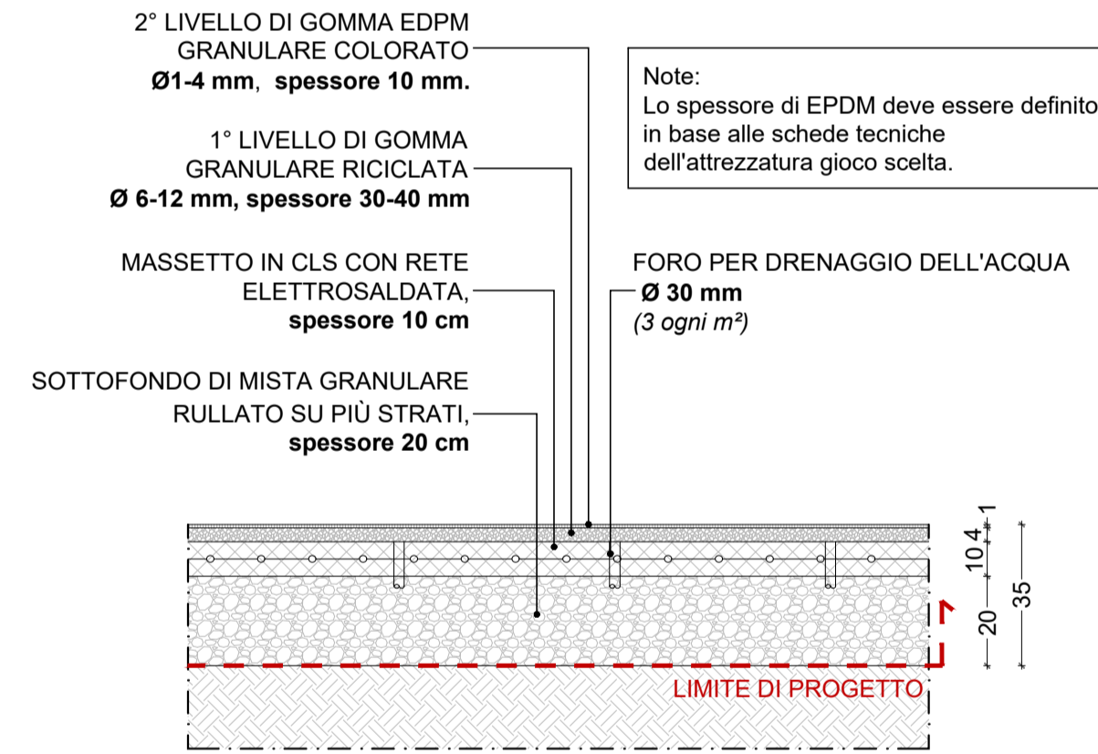
T7 Tipologico 7: Pavimentazione in gomma antitrauma scala 1:20
