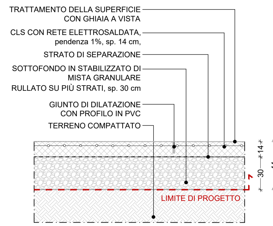
T1 Tipologico 1: CLS architettonico scala 1:20
