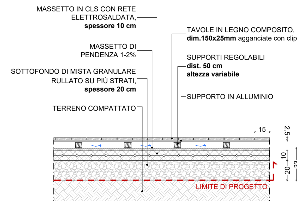
T8 Tipologico 8: Pavimentazione in legno composito scala 1:20
