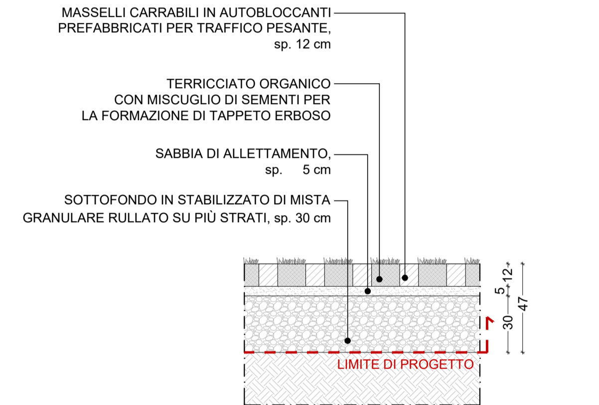
T6 Tipologico 6: Pavimentazione in prato armato scala 1:20
