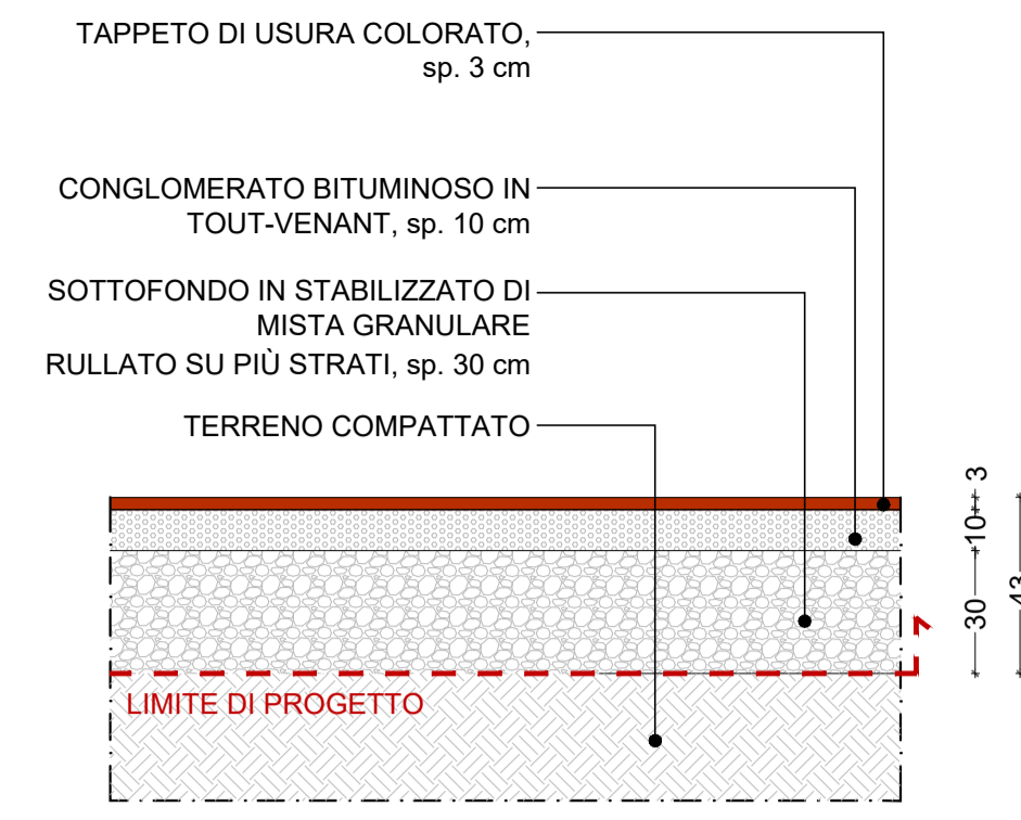
T5 Tipologico 5: Pavimentazione in asfalto colorato scala 1:20
