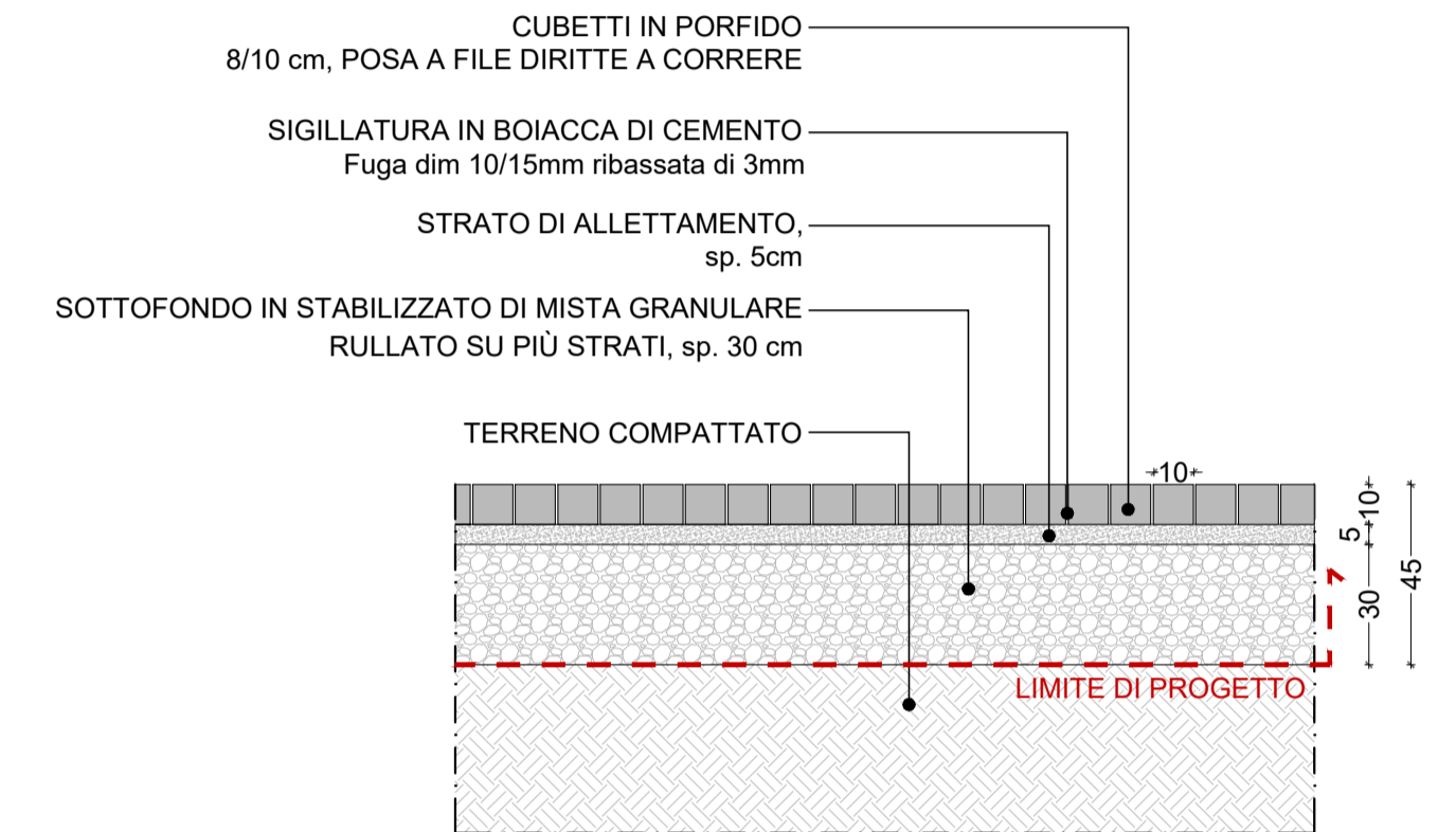
T10 Tipologico 10: Pavimentazione in cubetti (pedonale) scala 1:20
