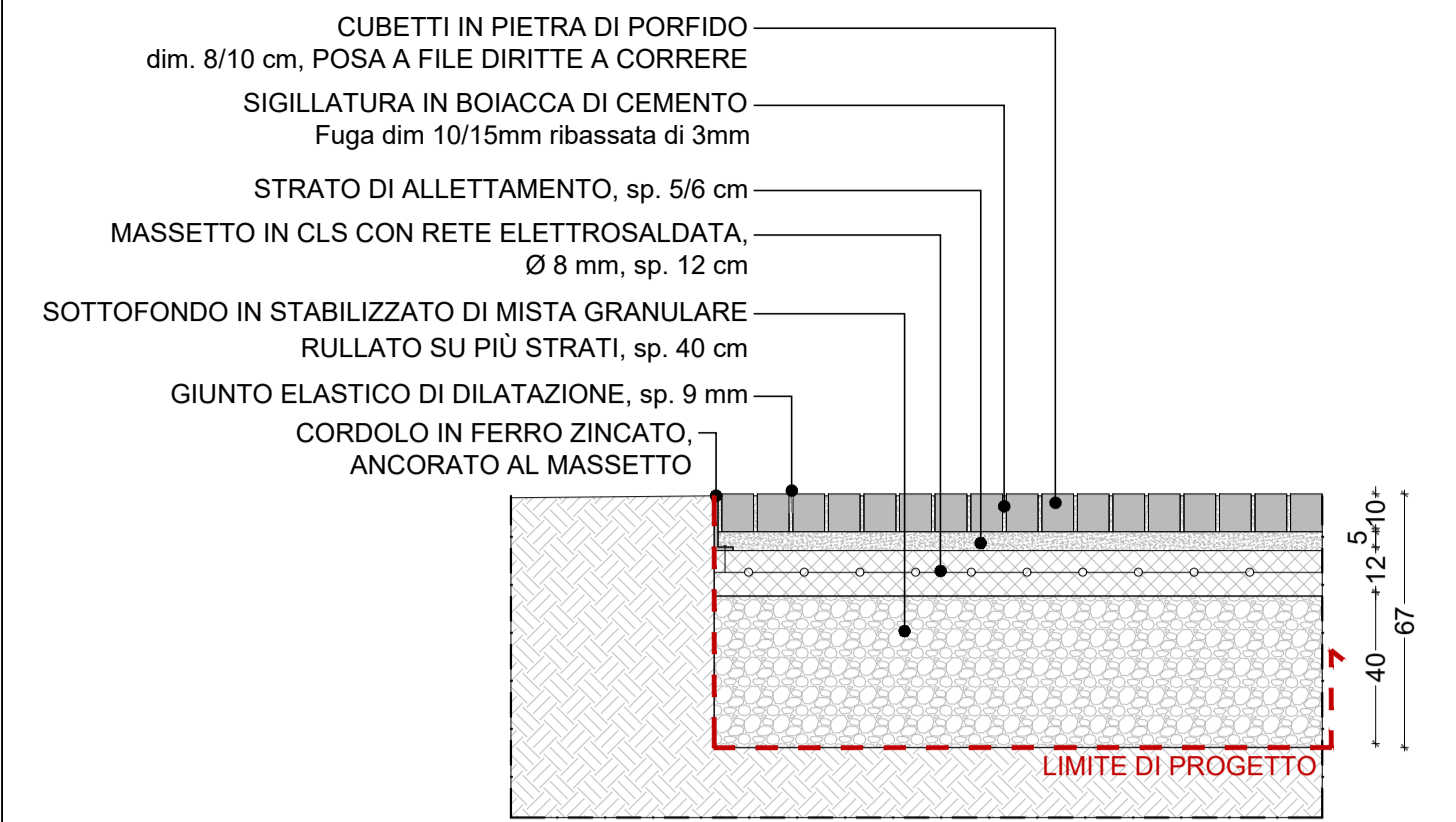
T9 Tipologico 9: Pavimentazione in cubetti (carrabile) scala 1:20
