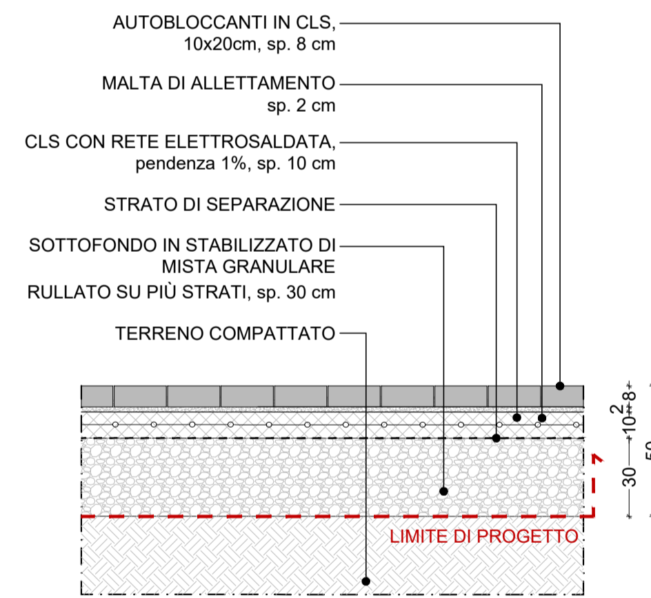
T3 Tipologico 3: Pavimentazione in autobloccanti (carrabile) scala 1:20
