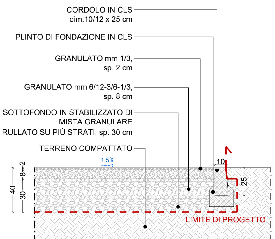
T4 Tipologico 4: Pavimentazione in calcestre scala 1:20
