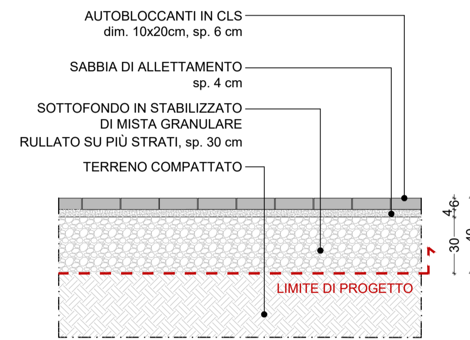
T2 Tipologico 2: Pavimentazione in autobloccanti (pedonale) scala 1:20
