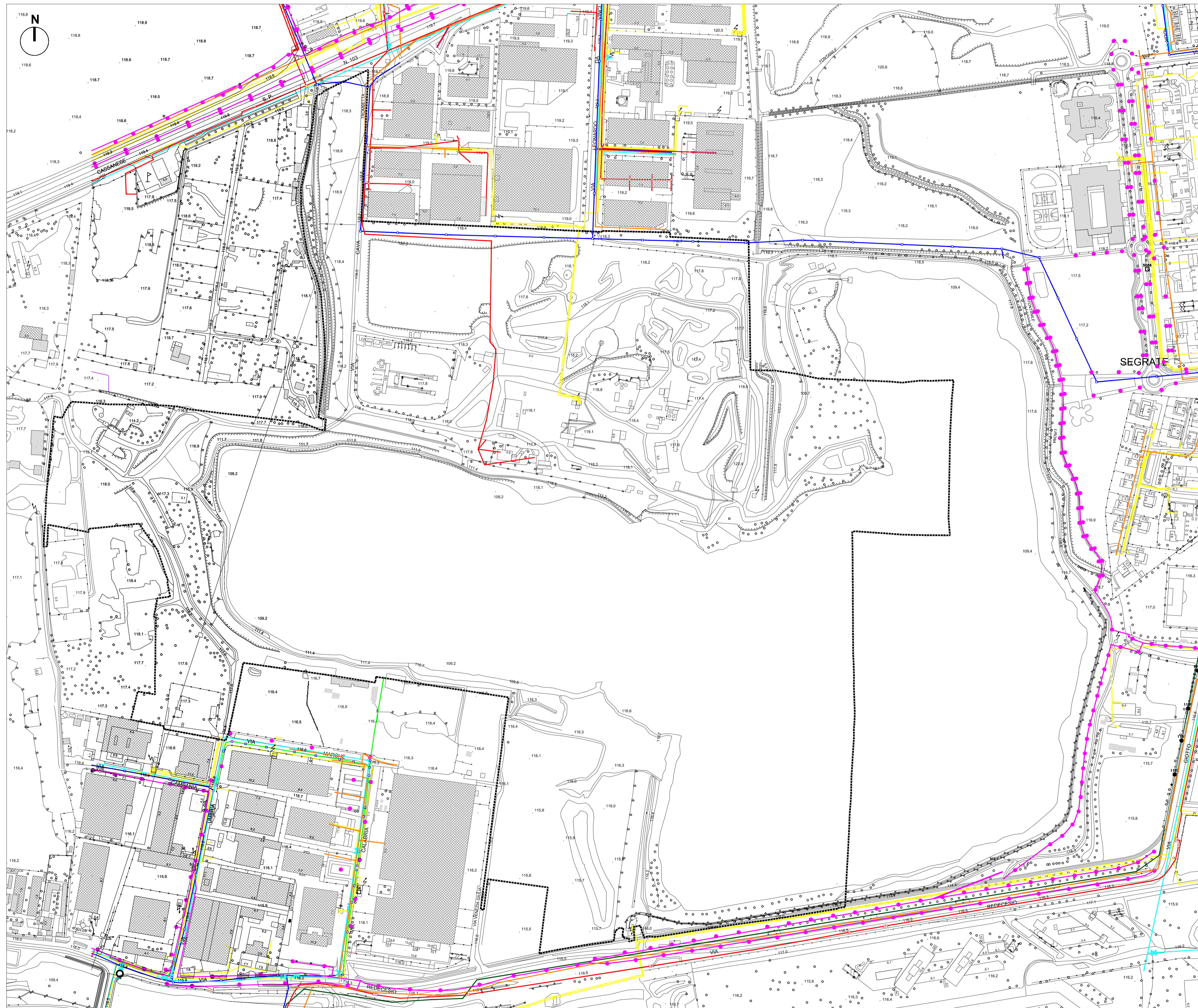
Planimetria generale, rete dei sottoservizi esistenti - scala 1:2000
